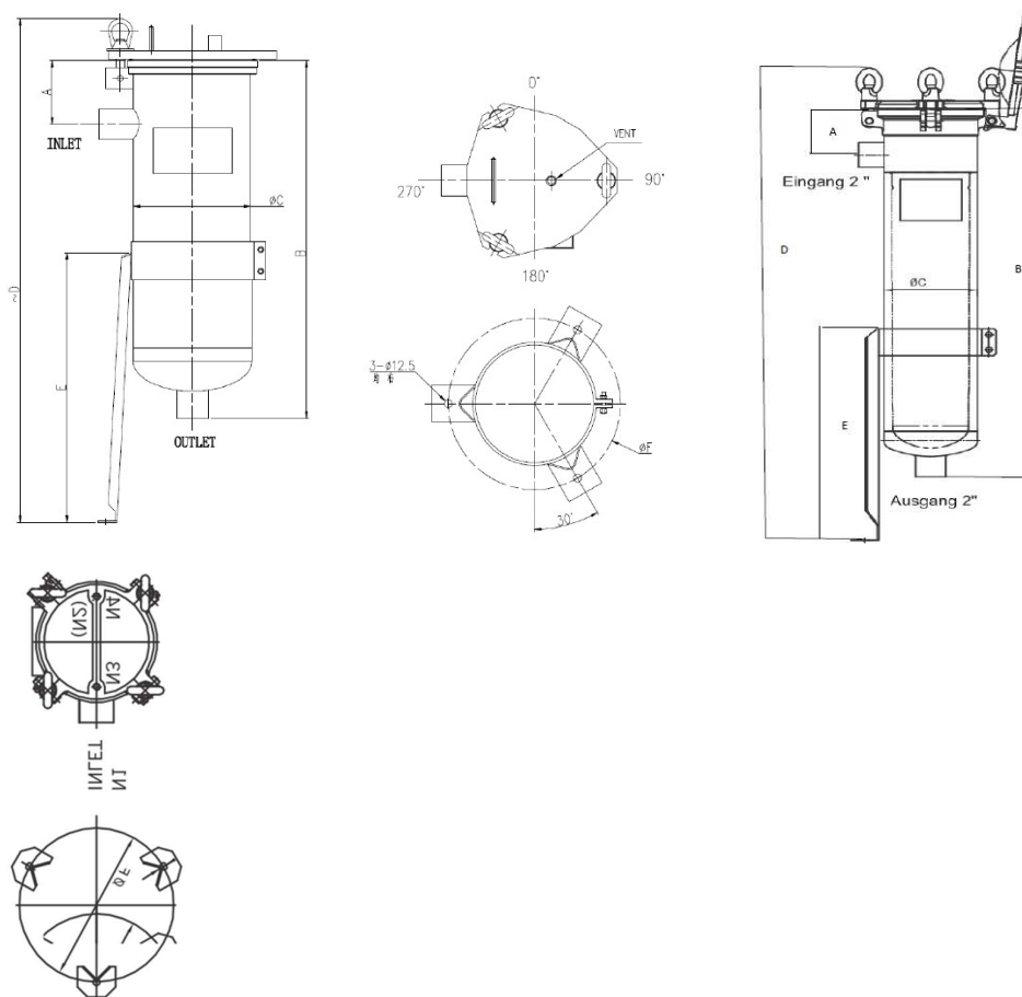
Abbildung 1: Abmessungen Beutelfilter
